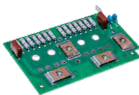
Плата диодная модуля СМ в сборе с радиатором
